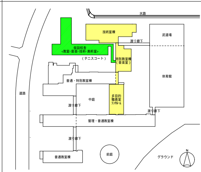
4期工事：多目的・職員室・ラウンジ + 音楽・技術室棟
