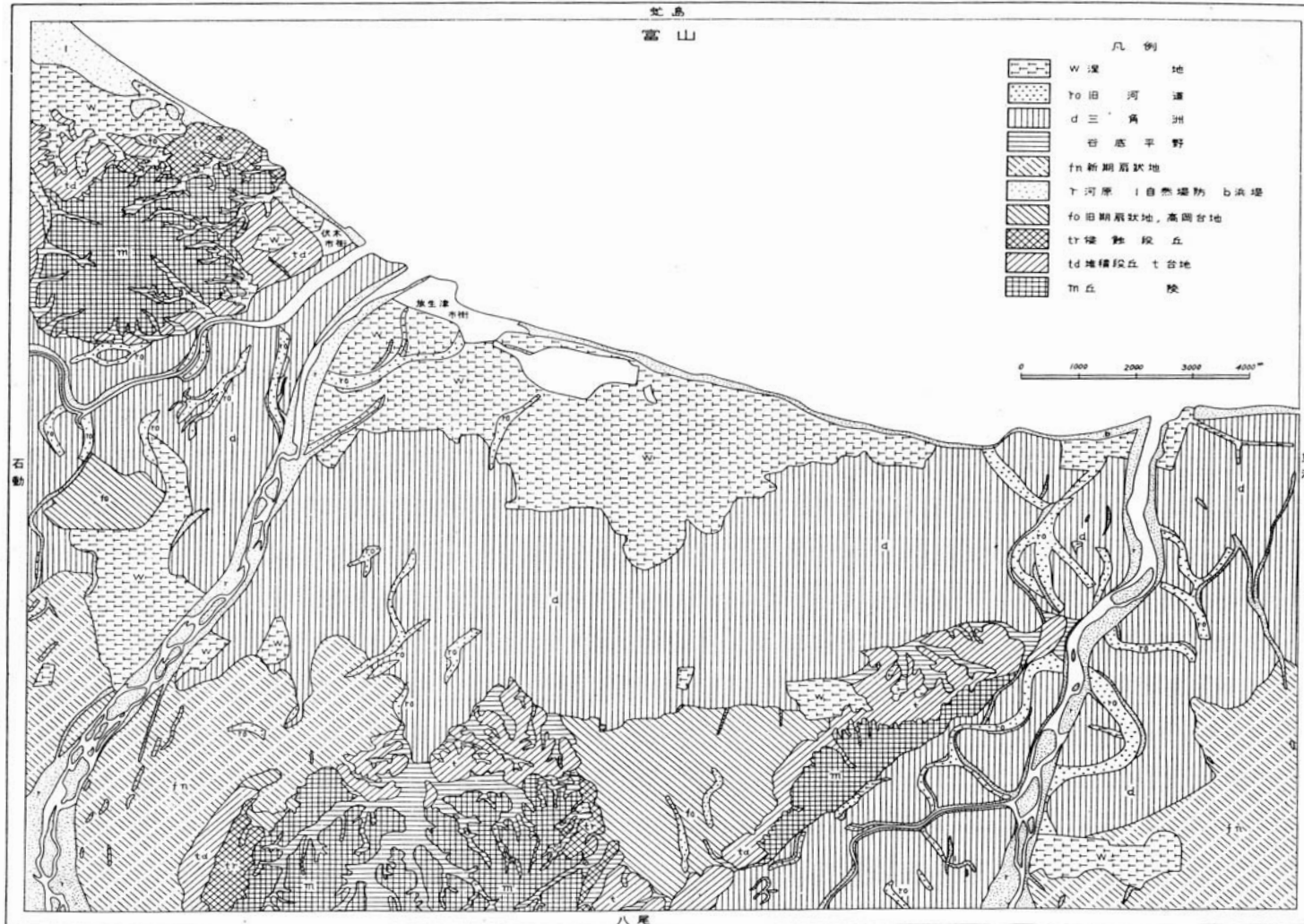
射水地区の微地形分類図
