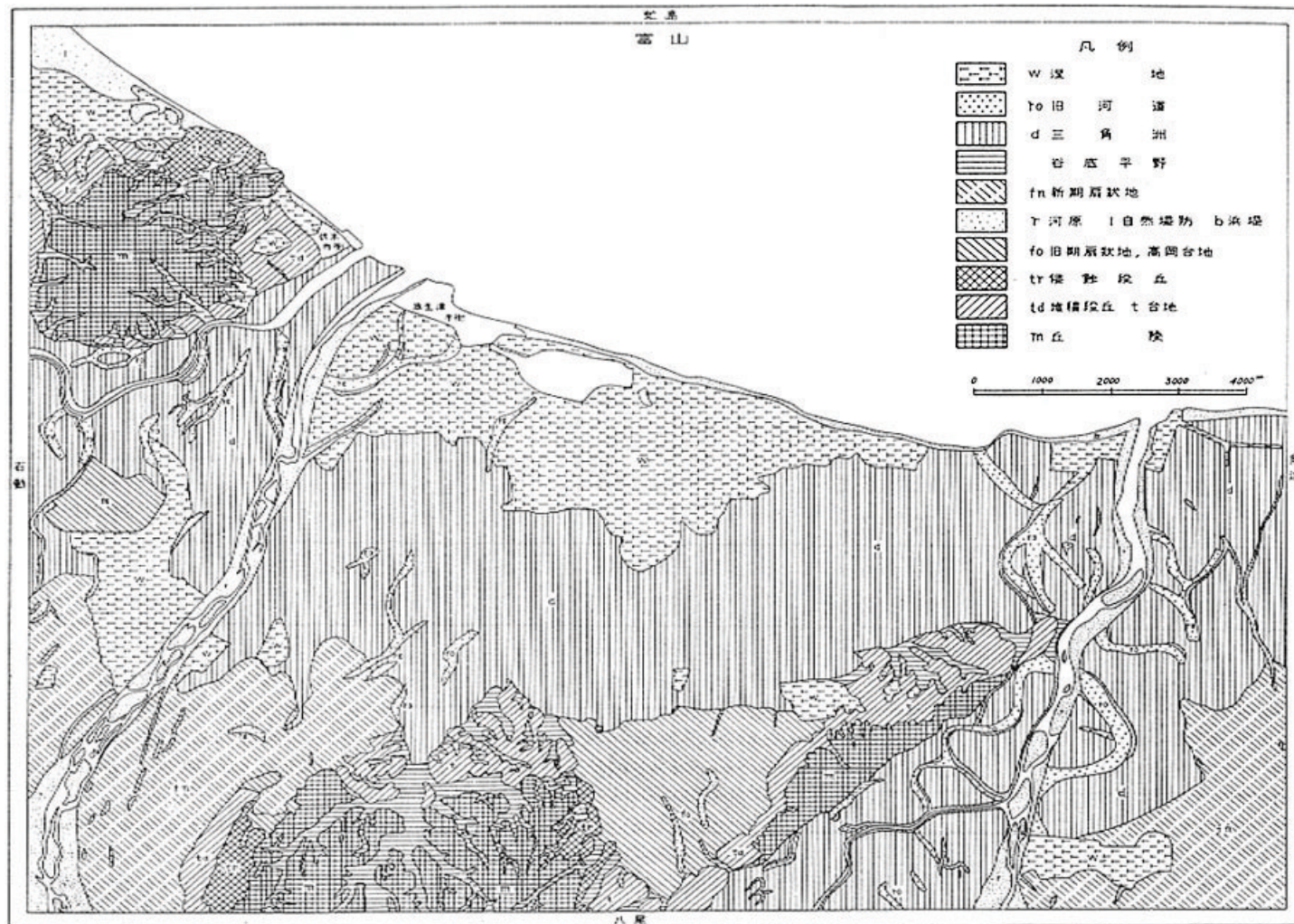
射 水 地 区 の 微 地 形 分 類 図
