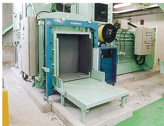
プラ・紙容器包装圧縮梱包機 プラスチックや紙容器を圧縮し梱包します。
