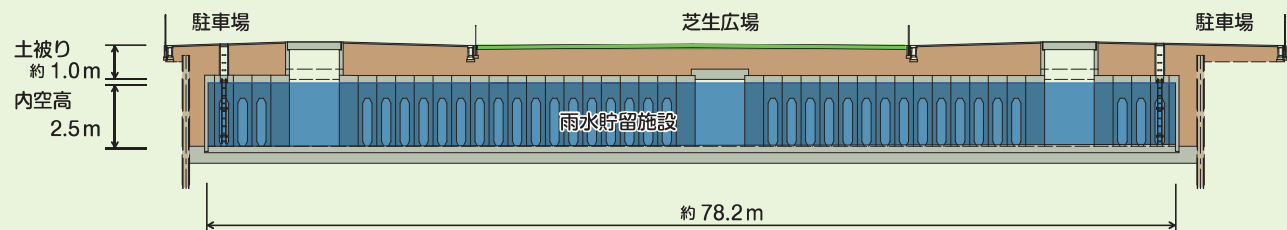
施設断面図 (A-A')
