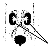
腎臓
