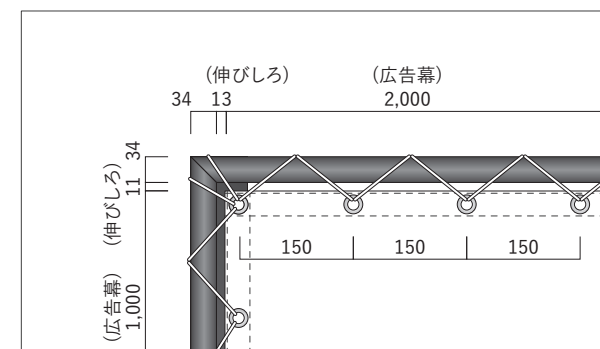
【拡大図 S=1/10】
