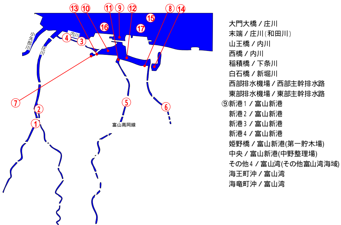
図4-1-1. 環境基準点の位置図
