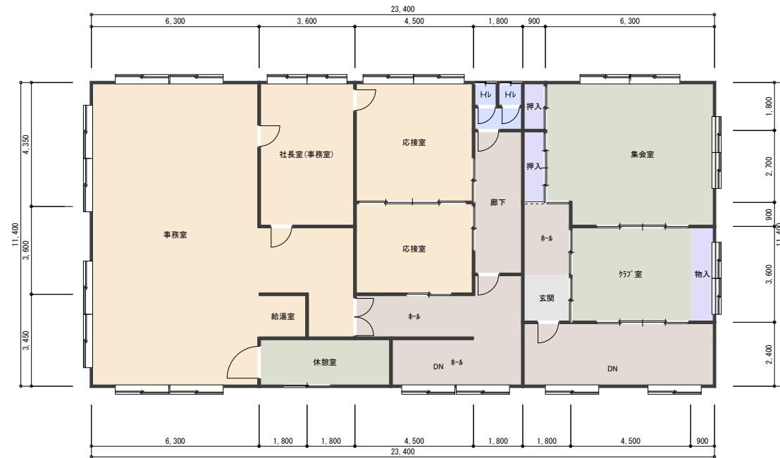
2階 縮尺 1/200
