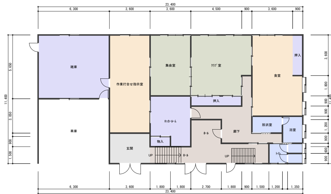
1階 縮尺 1/200
