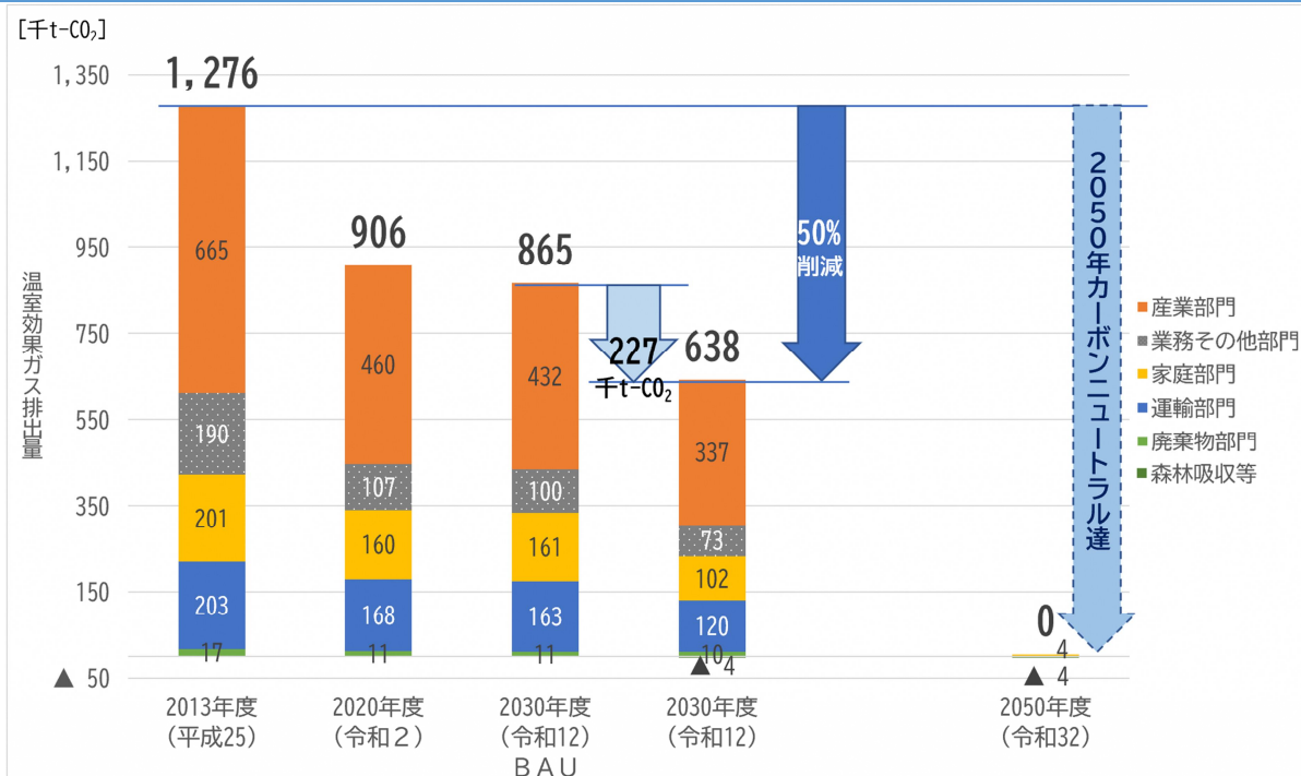
図 4-2 本市における温室効果ガス排出量の目標及び削減率
