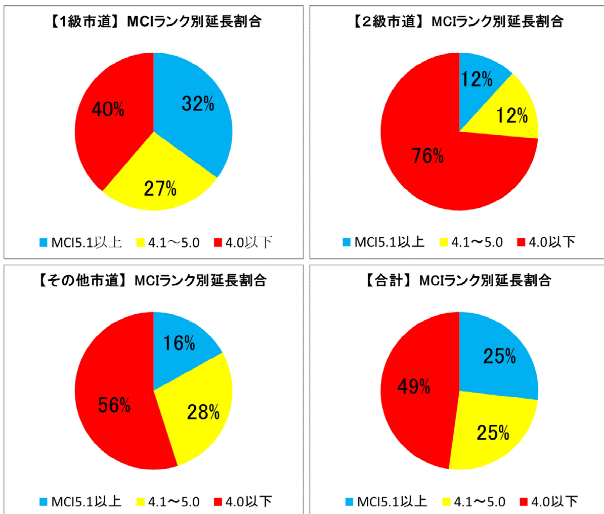
図-1 MCI ランク別延長割合
